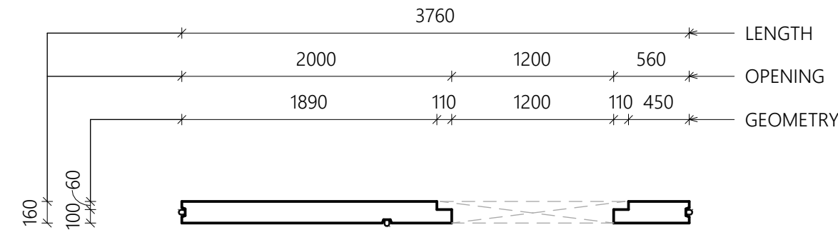
4 SECTION 1 : 40
