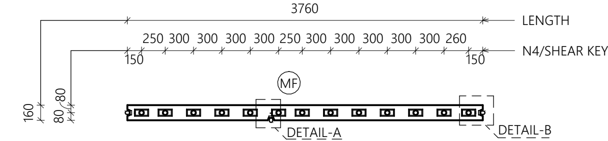
3 SECTION 1 : 40
