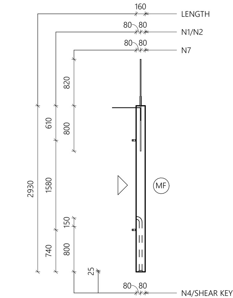
2 SECTION 1 : 40
